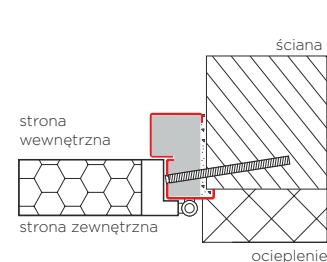
drzwi zewnętrzne otwierane na zewnątrz ościeżnica Termo ODS56
