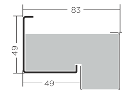
ościeżnica Termo ODS68 asymetryczna
