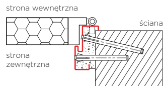
drzwi wewnętrzne otwierane do wewnątrz ościeżnica PU/UNI56
