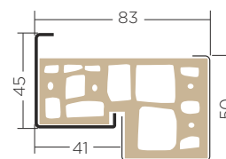
ościeżnica SK56 stalowo-kompozytowa asymetryczna
