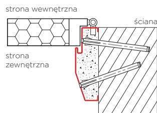
drzwi wewnętrzne otwierane do wewnątrz ościeżnica PD56
