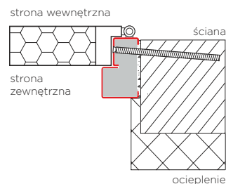
drzwi zewnętrzne otwierane do wewnątrz ościeżnica Termo ODS56
