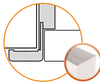
drzwi bezprzylgowe
